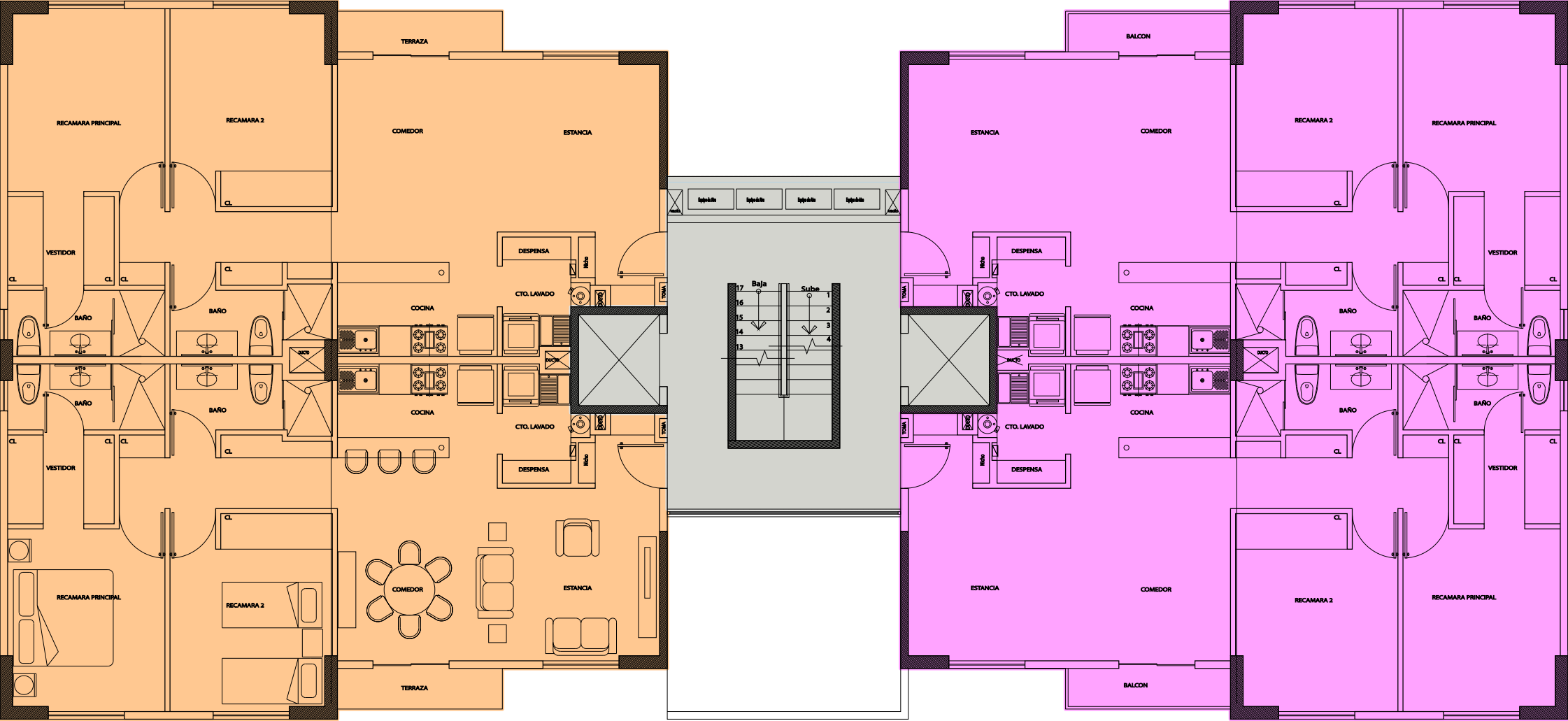
PLANTA NIVEL 1
