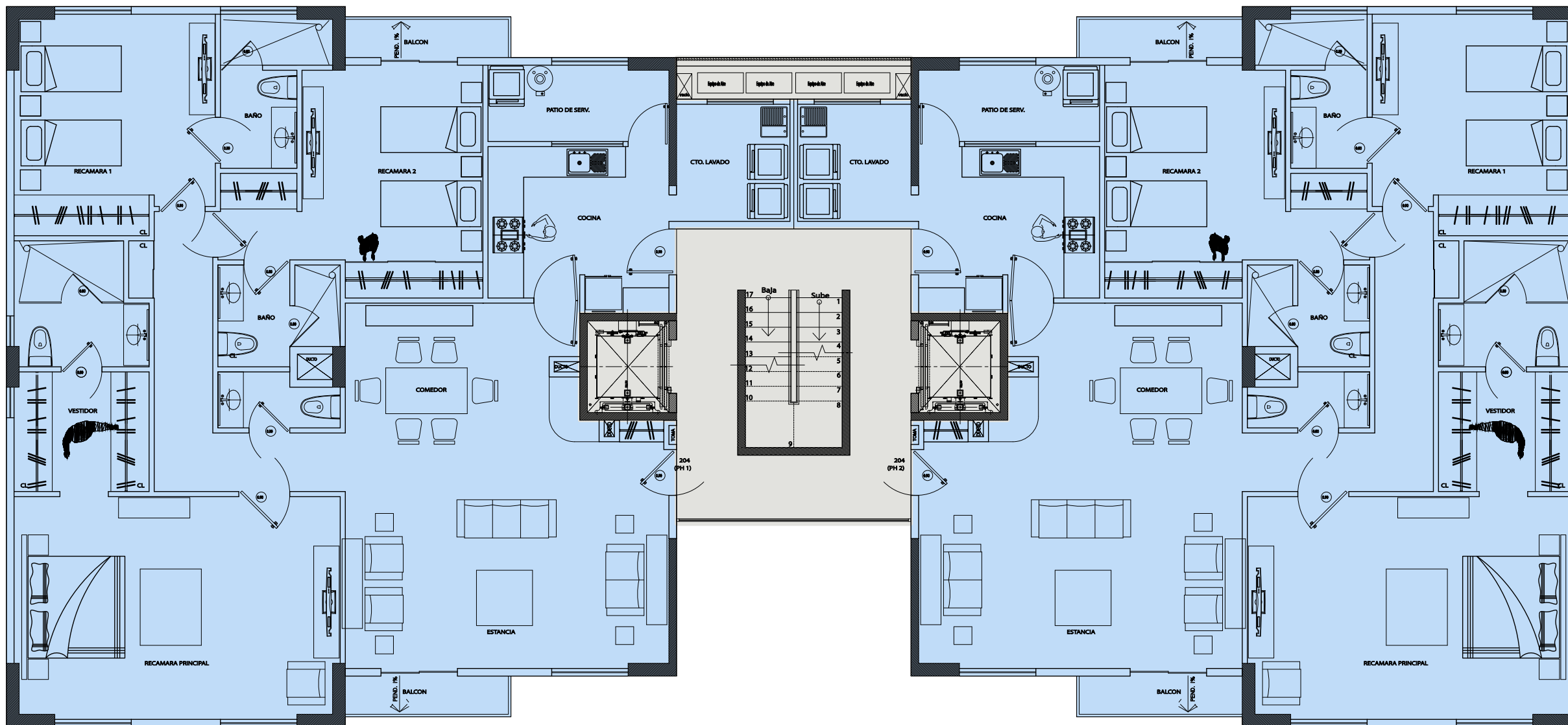
PLANTA 6° AL 9° PISO
